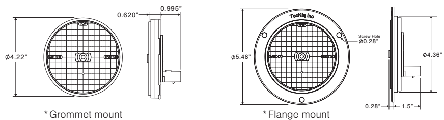
* Grommet mount
