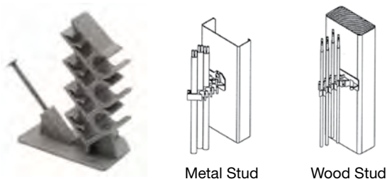
Metal Stud
